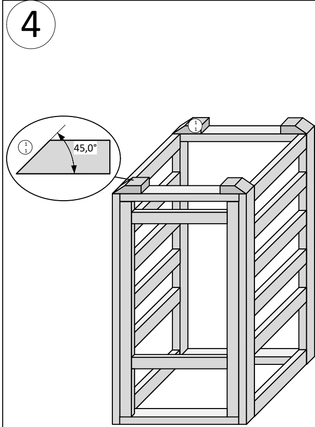
Vyrobte a připevněte šikmé hranoly pro uchycení střechy
