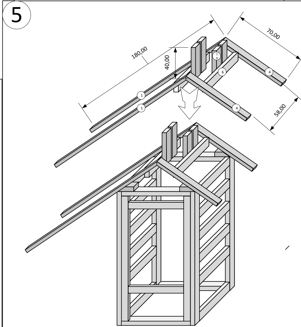
Smontujte střechu a přišroubujte na boudu
